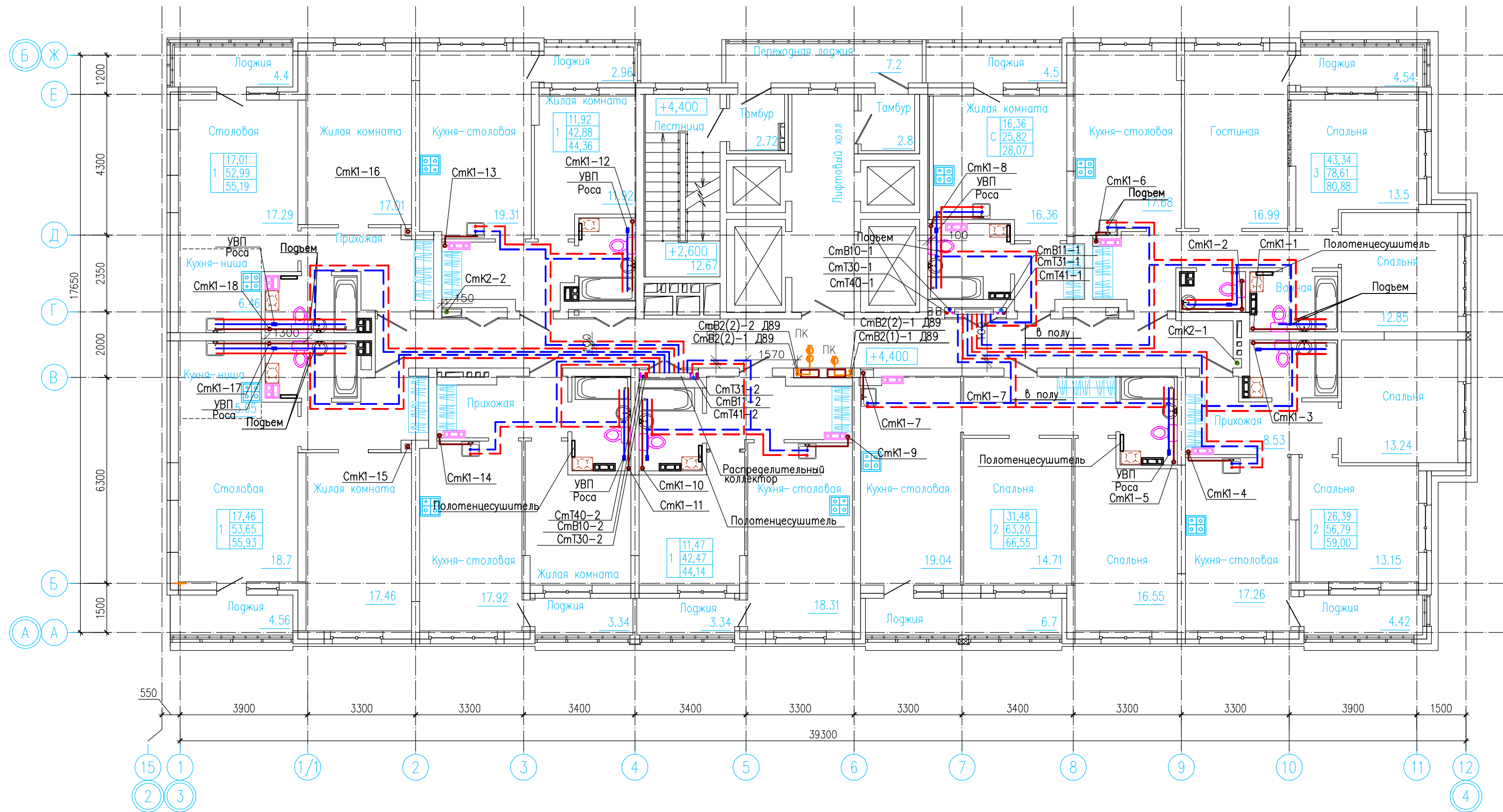
Фрагмент плана 2 этажа
